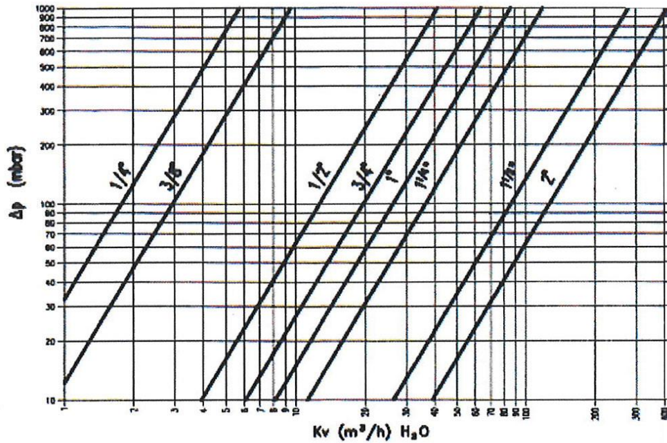
Druckverlustdiagramm
